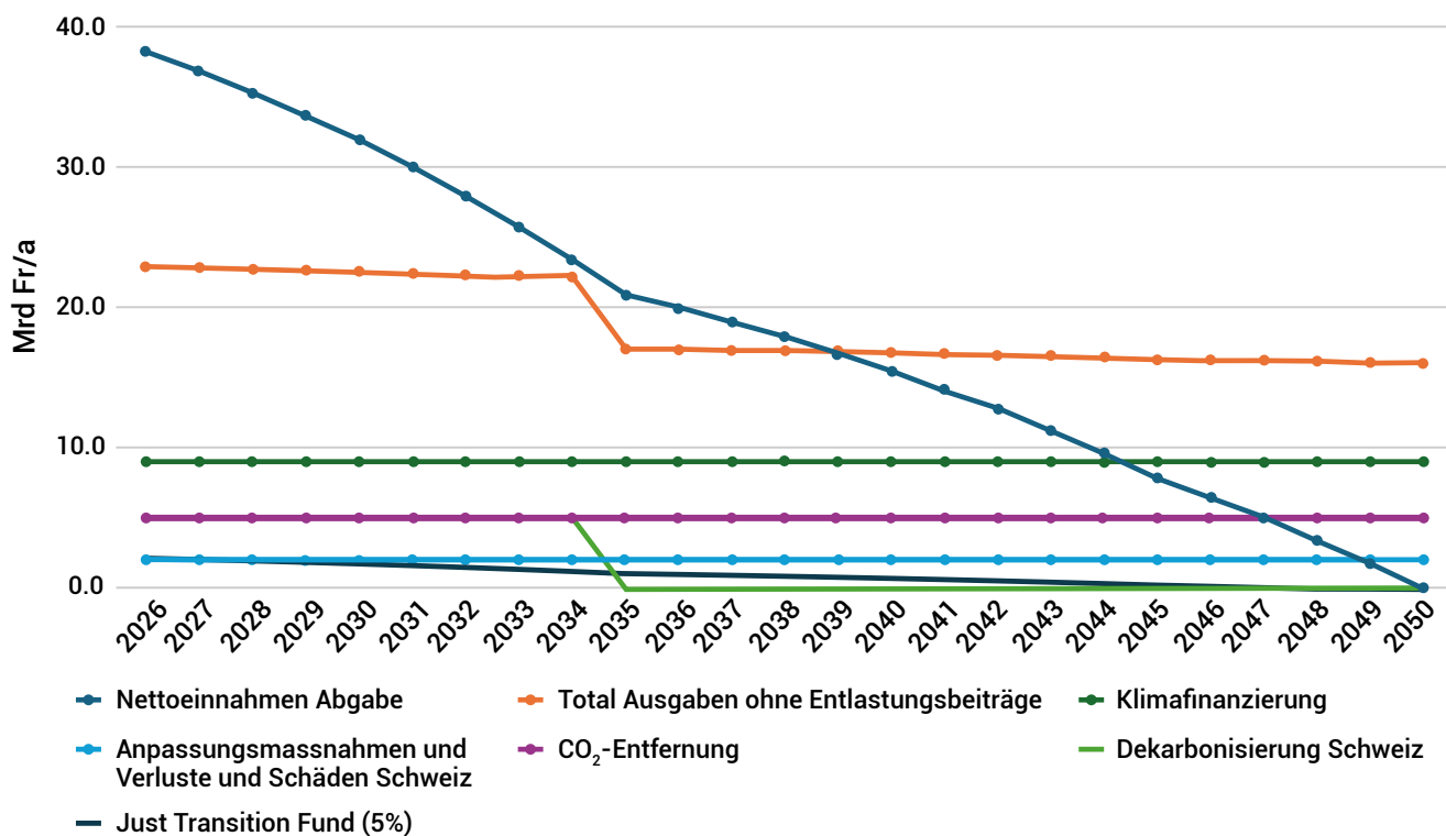
Abbildung 4: Geschätzter Verlauf der Einnahmen aus der Treibhausgasabgabe und geplanten Ausgaben aber noch ohne nötige Entlastungsbeiträge für Haushalte in bescheidenen finanziellen Verhältnissen. Quelle: Klima-Allianz.
