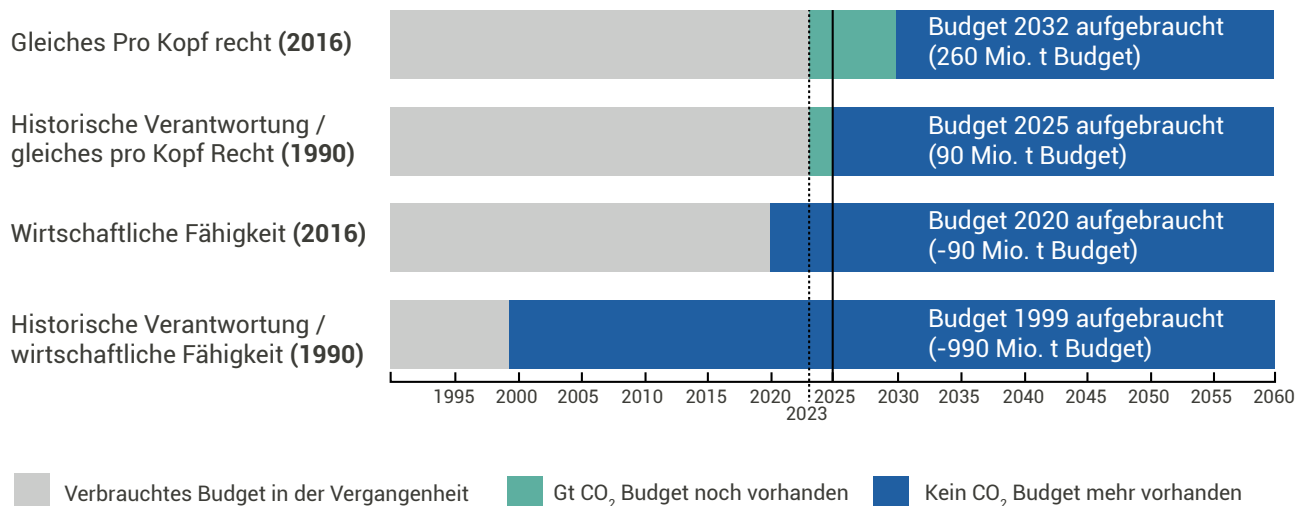
Abbildung 2: Ansätze zur Aufteilung des noch verfügbaren globalen CO 2 -Budgets (1.5°C / 50% Wahrscheinlichkeit) Quelle: Pelz et al 2025
