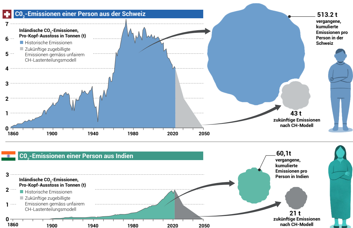
Abbildung 1: Der Vergleich Schweiz gegen Indien zeigt auf: die Aufteilung vom CO 2 Budget, wie es die Schweiz vorschlägt ist nicht fair. Quelle Infografik.ch
